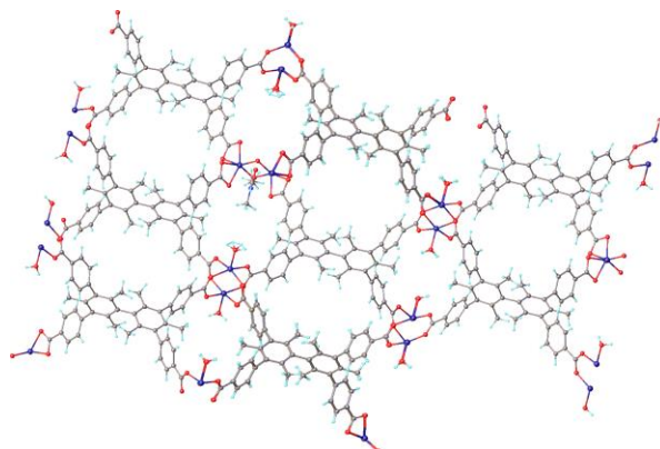
Fig. 8b. Proiecția structurii cristaline a complexului de cobalt.
