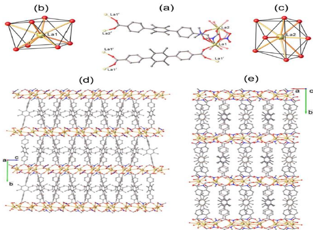
Fig. 5. (a) O vedere a părții asimetrice care prezintă modul de coordonare al atomilor de La. (b) poliedrul de coordonare al atomului de La1; (c) poliedrul de coordonare al atomului La2; (d) o vedere parțială a împachetării în cristal de-a lungul axei a ; (e) o vedere parțială a împachetării în cristal de-a lungul axei c .
