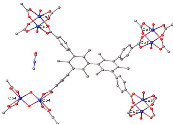
Fig. 8a. Fragment al rețelei coordinative din complexul de cobalt.
