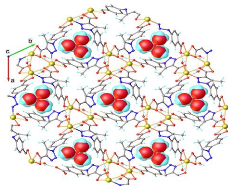
Fig.7. Asamblarea parțială a structurii cristaline a {[CdL(H 2 O)]·0.5H 2 O}n de-a lungul axei c.
