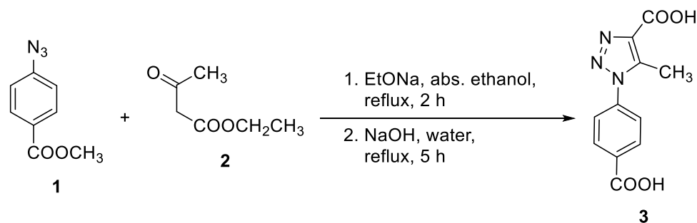
Schema 1. Sinteza ligandului H_2L ( 3 ) prin cicloadiția Dimroth.
