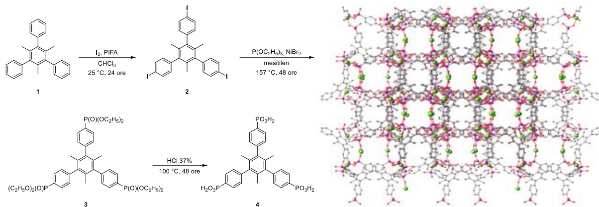
Fig. 9. Schema de sinteză a acidului mezitiltrifenilfosonic. Fig 10. Structura complexului polimeric
