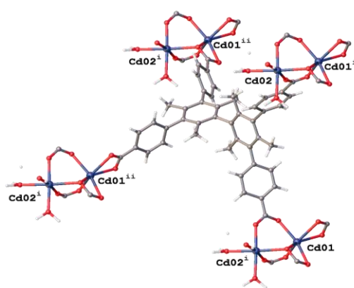
Fig. 6 Compusul TCMES-Cd 2 (4)
