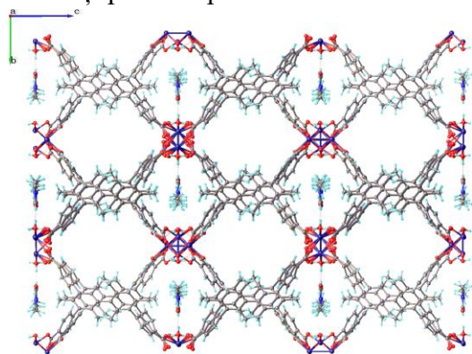
Fig. 3. Complexul TCMES-Zn 7 ( 1 )
