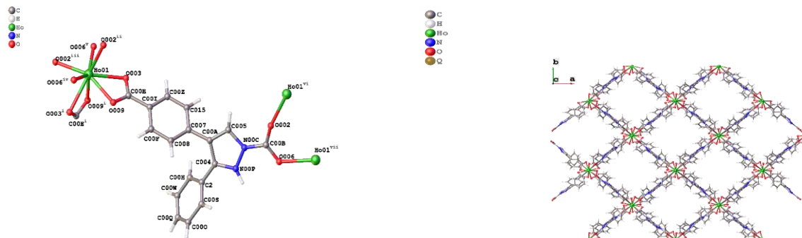
Figura 8. Structura compusului LP-Ho (mod de coordonare și orientare după axa c)
