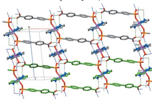
Figura 12. Legăturile de hidrogen intra si inter-banda sunt prezentate ca linii intrerupte în verde și, respectiv, albastru; intramolecular.
