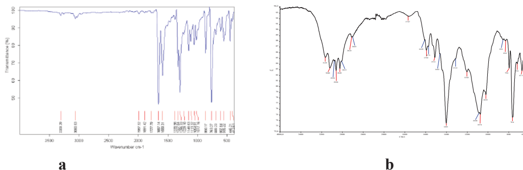
Рис. 1. ИК-спектр 1,4-ПДАН, полученного методом окислительной полимеризации без ДДА (а); с ДДА (b).
