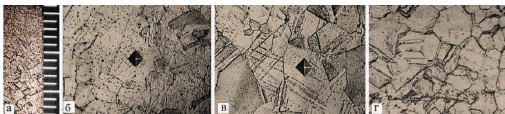
Рис. 1. Сталь AISI 316L, сухое трение «металл/металл»: AISI 316L/сталь СтЗсп, вид на плоскости в сечении, длительность трения t = 1 час; а– микроструктура образца при небольшом увеличении, сверху поверхность трения, 1 деление масштабной линейки равно 10 мкм; б-г – вид микроструктуры образца и отпечатков твердости, нанесенных на разных расстояниях от поверхности трения; горизонтальная сторона каждого кадра равна 180 мкм.
