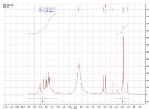
Рис. 5. 1 H-ЯМР спектр поли-(1,4-ДАНa).
