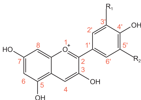
Figura 4. Structura chimică generală a unor antociani: Cianidina ( R_1=OH ; R_2=H ); pelargonidina ( R_1=R_2=H ); delphinidina ( R_1=R_2=OH ); peonidina ( R_1=OCH_3 ; R_2=H ); petunidina ( R_1=OH ; R_2=OCH_3 ); malvidina ( R_1=R_2=OCH_3 ).
