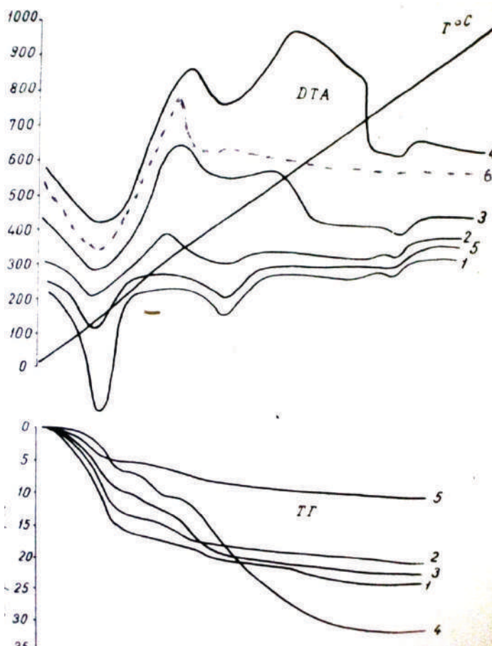
Рис.3. Дериватограммы образцов монтмориллонитовых глин модифицированных алкиламмониевыми катионами: 1 – ларгуцкий бентонит, 2 – ларгуцкий бентонит 0,001N, 3 – ларгуцкий бентонит 0,01N, 4 – ларгуцкий бентонит 0,1N, 5 – ларгуцкий бентонит Na – форма, 6 - АБДМ
