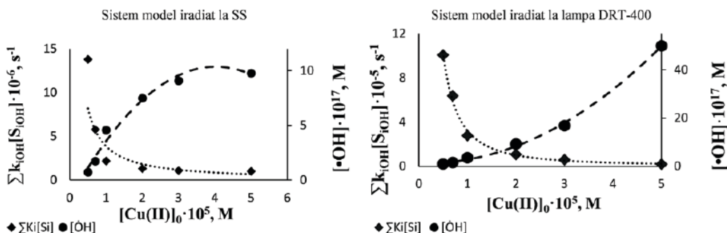
Fig. 5. Variația capacității de inhibiție și concentrației radicalilor OH în funcție de concentrația ionilor de Cu(II), la diferite surse de iradiere, [PNDMA]_0 = \text{const} = 2,0 \cdot 10^{-5} \text{ M} , [H_2O_2]_0 = \text{const} = 1 \cdot 10^{-2} \text{ M} , [CNCbl]_0 = \text{const} = 1 \cdot 10^{-6} \text{ M} pH=6,2, t=25 \text{ }^\circ\text{C} [date proprii]
