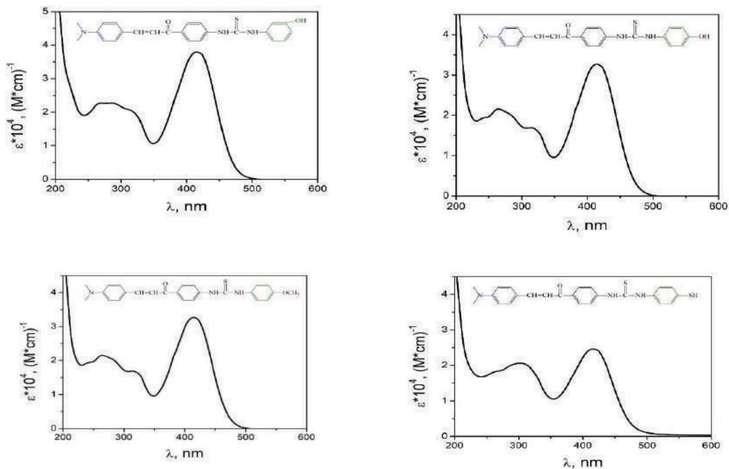
Fig. 2. Spectrele de absorbție UV-Vis separate al compușilor 1b-e
