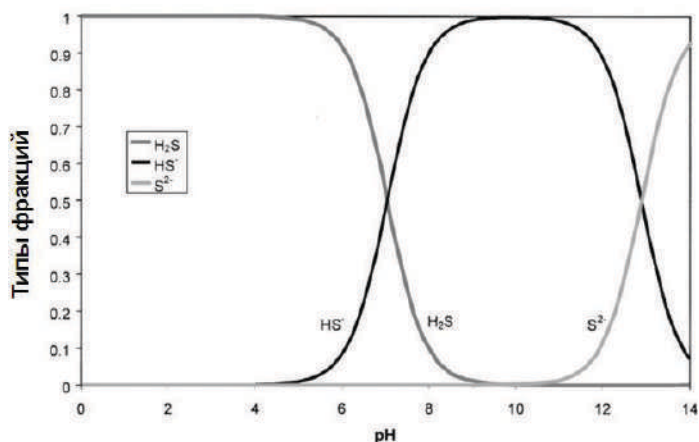
Рис.2. Диссоциация сероводорода [9].
