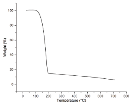
Рис. 4. ТГ поли-(1,4-ДАНa).
