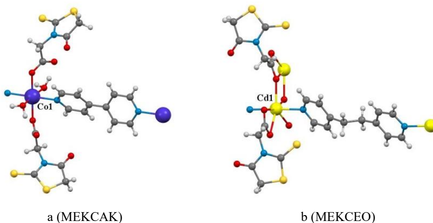
Figura 5. Structura fragmentelor polimerilor coordinativi cu Rda și liganzi suplimentari din clasa bipiridinelor: a) a polimerului de Co(II); b) a polimerului de Cd(II).
