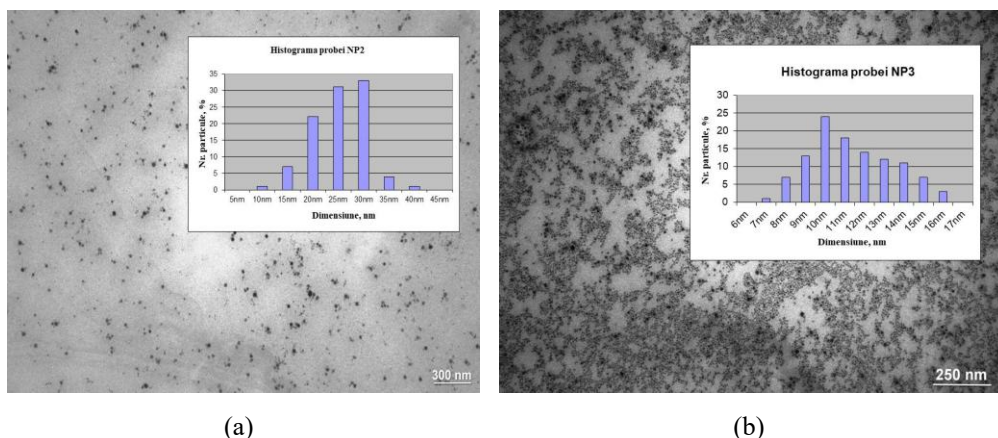
Figura 4. Imagini MET și histogramele distribuției particulelor după dimensiune pentru probele NP2 (a) și NP3 (b)
