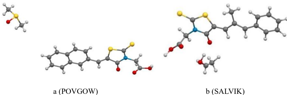
Figura 11. Structura derivaților rodaninei cristalizați cu molecule de solvatare având formula generală Rda-(C5)-R1 : a) R1- naftilmetilen; b) R1 - 2-metil-3-fenilprop-2-enilidene (epalrestat).
