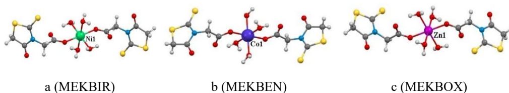
Figura 4. Structura moleculară a compușilor cu Rda: a) a complexului de Ni(II); b) a complexului de Co(II); c) a complexului de Zn(II).
