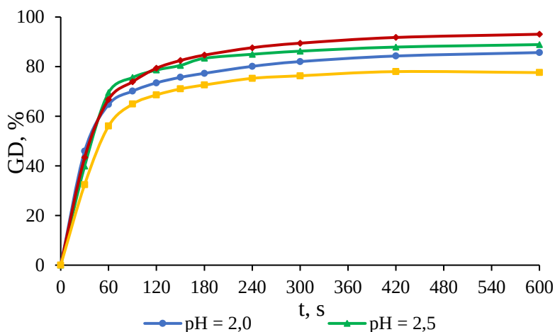
Figura 5. Dependenta gradului de degradare a CFX de timp în sistemul foto-Fenton la diferite valori ale pH-ului
