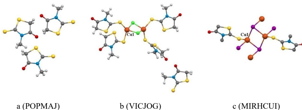
Figura 2. a) Structura moleculară a 3-metil-N-rodaninei; b) structura moleculară a complexului dinuclear de Cu(II) cu acest ligand; c) Fragment din structura polimerului coordinativ unidimensional de Cu(II).
