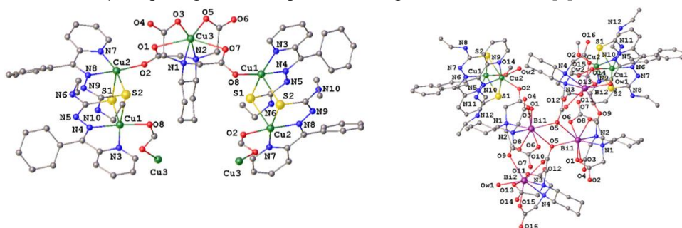
Figura 4. Structura complexului a) homometalic \{[Cu_2(BzPyTSC-4Et)_2Cu(cdta)] \cdot 3.95H_2O\}_n și b) heterometalic \{[Cu_2(BzPyTSC-4Et)_2Bi_2(cdta)_2(H_2O)_2] \cdot 13.25H_2O\}_n [9]
