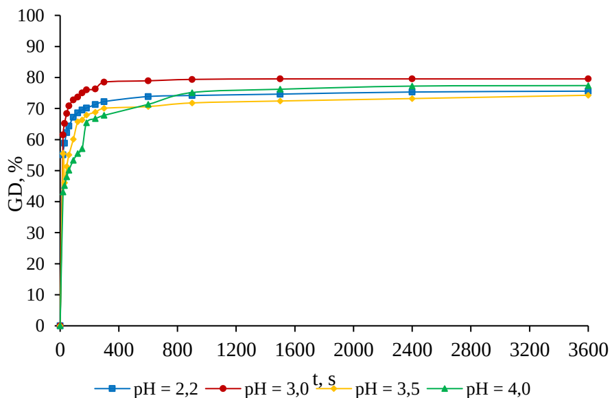
Figura 4. Dependența gradului de degradare a CFX de timp în sistemul Fenton la diferite valori ale pH-ului
