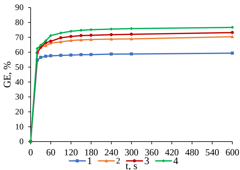
Figura 8. Dependența GD = f(t) pentru diferite concentrații ale CFX în sistemul Fenton: 1 - 2,0 \cdot 10^{-5} M; 2 - 3,0 \cdot 10^{-5} M; 3 - 3,5 \cdot 10^{-5} M; 4 - 4,0 \cdot 10^{-5} M
