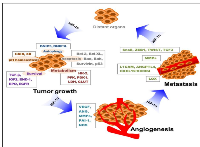
Figura 4. Rolul HIF-1 în creșterea tumorală, angieneză și metastazăre [21].
