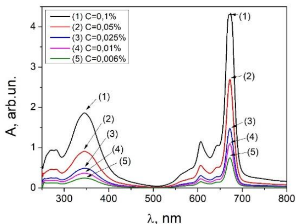
Figura 2. Spectrele de absorbție ale AM-PcZn
