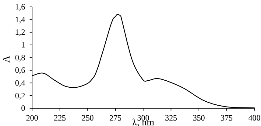
Figura 2. Spectrul electronic de absorbție a ciprofloxacinei în soluție apoasă ( [\text{CFX}] = 3,24 \cdot 10^{-5} M; \text{pH} = 3,0 )
