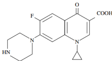
Figura 1. Formula structurală a ciprofloxacinei [15, p. 148]
