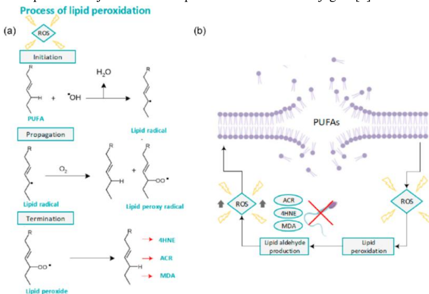
Figura 1. Reprezentarea schematică a cascadei peroxidării lipidice structurată în trei etape fundamentale și generarea alchidelor lipidice electrofile rezultate din degradarea oxidativă [13].
