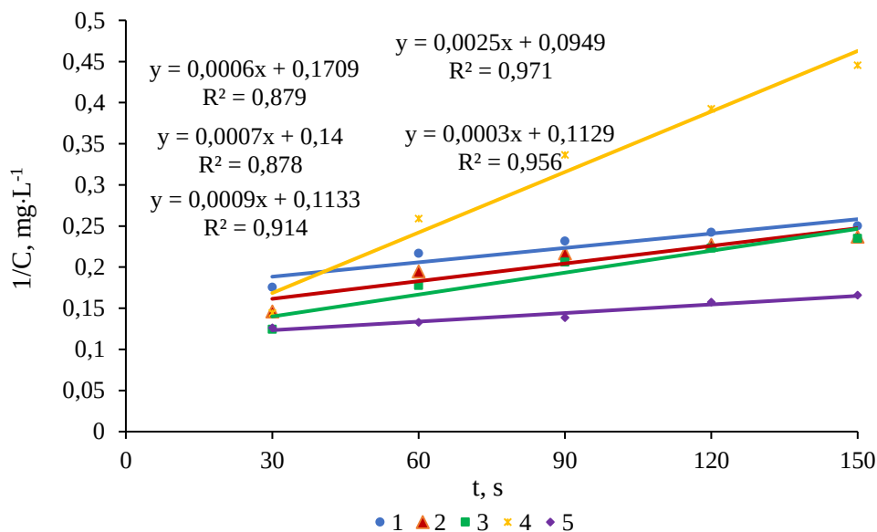
Figura 11. Dependențele 1/C = f(t) pentru degradarea CFX în sistemul foto-Fenton la diferite concentrații ale CFX: 1 – 2,0 \cdot 10^{-5} M; 2 – 2,5 \cdot 10^{-5} M; 3 – 3,0 \cdot 10^{-5} M; 4 – 3,5 \cdot 10^{-5} M; 5 – 4,0 \cdot 10^{-5} M
