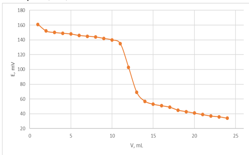
Figura 4. Curba integrală de titrare a soluției model ce conține ioni de zinc cu soluție de hidroxid de sodiu 0,1 mol/L, utilizând în calitate de electrod indicator EIS 2
