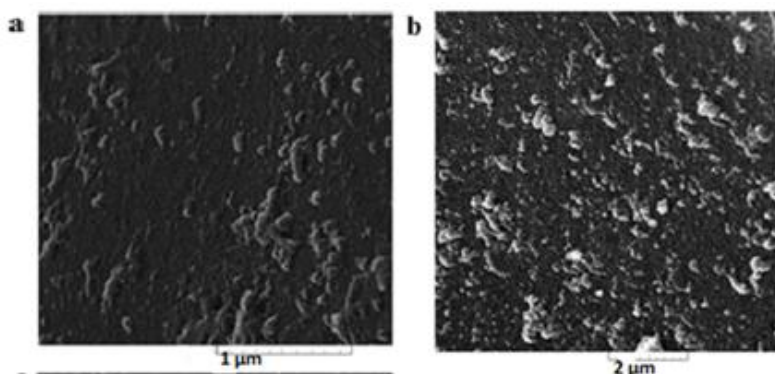
Figura 6. Imaginile SEM a Cr-jarozitului pe suprafața (a) și în volumul granulelor de polimer AV-17.
