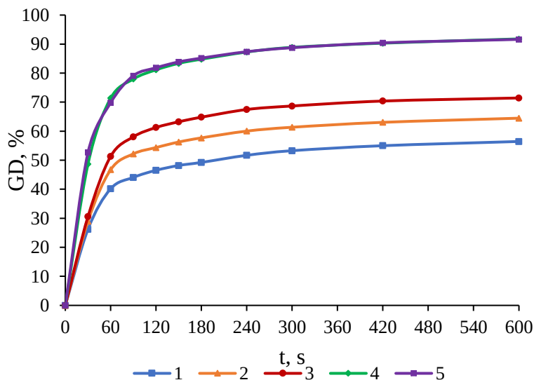
Figura 9. Dependența GD = f(t) pentru diferite concentrații ale CFX în sistemul foto-Fenton: 1 - 2,0 \cdot 10^{-5} M; 2 - 2,5 \cdot 10^{-5} M; 3 - 3,0 \cdot 10^{-5} M; 4 - 3,5 \cdot 10^{-5} M; 5 - 4,0 \cdot 10^{-5} M
