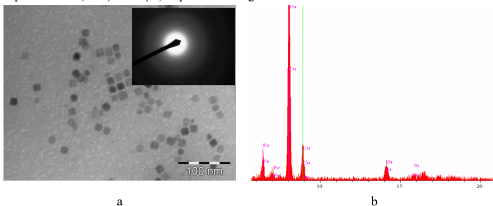
Figura 3. (a) Imaginea MET și difracția de electroni, (b) spectrul EDX ale probei NP1
