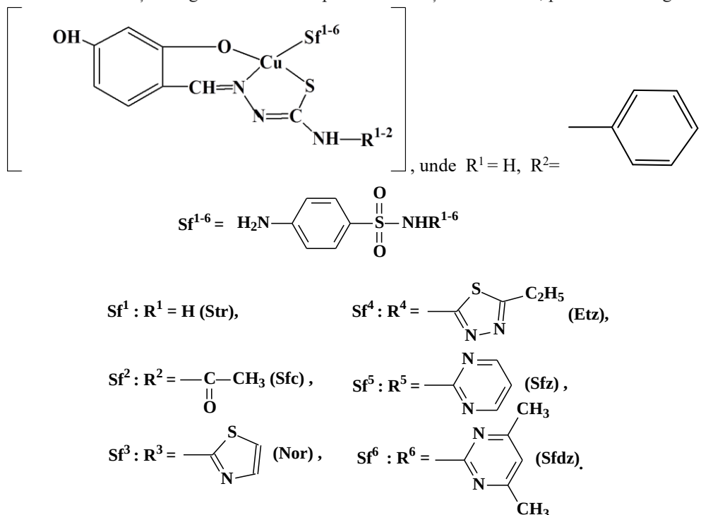
Figura 3. Schema distribuției legăturilor chimice în compuși coordinați
