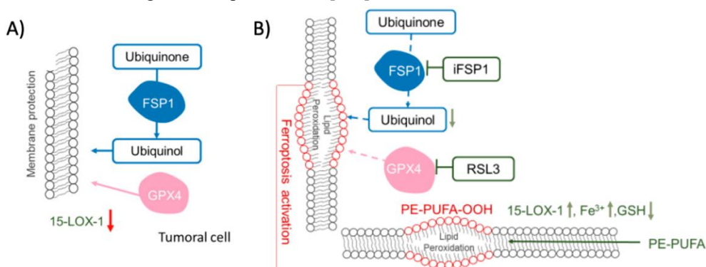
Figura 2. Mecanismele de protecție ale celulelor tumorale împotriva peroxidării lipidice prin intermediul sistemelor enzimatic glutatoni peroxidaza 4 și proteina 1 de suprimare a ferroptozei [1].
