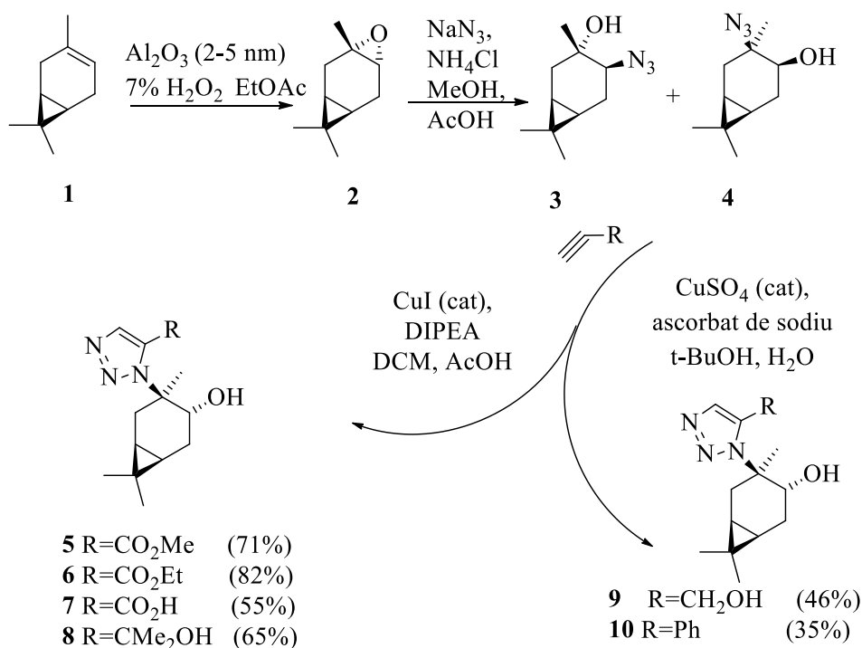
Figura 1. Schema de sinteză a 1,2,3-triazolilor din (+)-3-carenă
