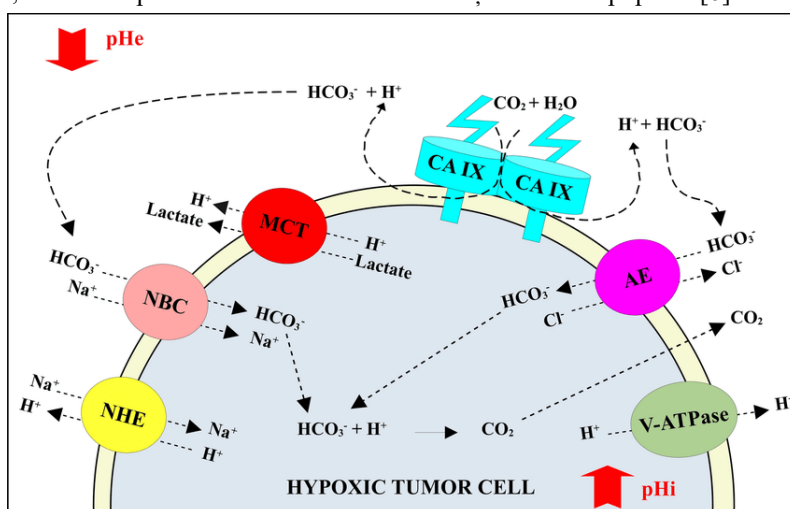
Figura 3. Modificări post-tranlaționale în anhidraze carbonice asociate tumorii [32].
