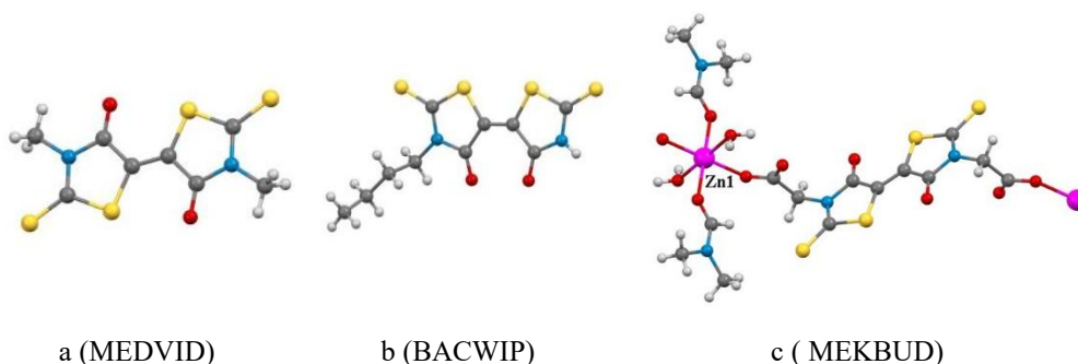
Figura 12. a) Structura uni derivat simetric al rodaninei cu formula \text{CH}_3\text{-N3-Rd-Rd-N3-CH}_3 ; b) Structura uni derivat asimetric al rodaninei cu formula \text{RdH-Rd-N3-C}_4\text{H}_9 ; c) Fragment din structura polimerului coordinativ al \text{Zn(II)} cu derivatul 5,5'-Rda-Rda.
