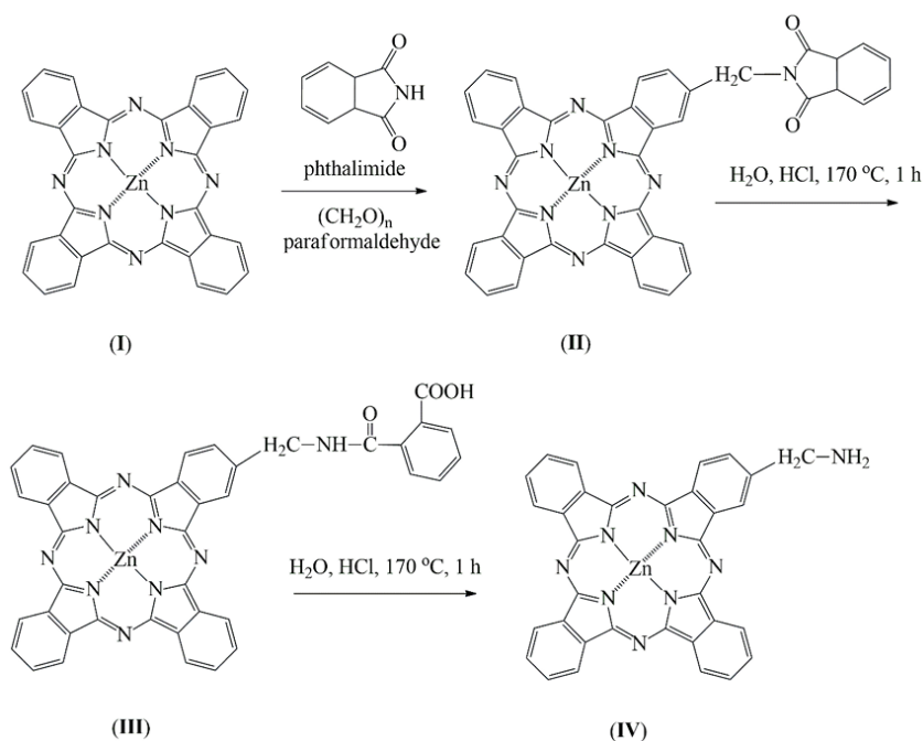
Schema 1. Schema de sinteză a AM-PcZn
