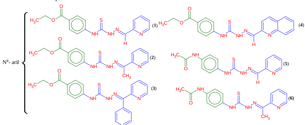
Figura 2. Formule de structură pentru tiosemicarbazonele 1-6, care conțin în poziția N 4 fragmentul aromatic
