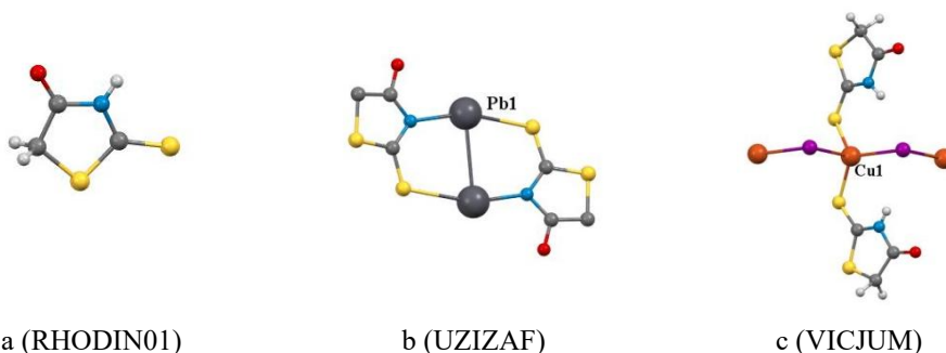
Figura 1. a) Structura moleculară a rodaninei; b) Structura moleculară a complexului dinuclear de Pb(II); c) Fragment din structura polimerului unidimensional de Cu(II).
