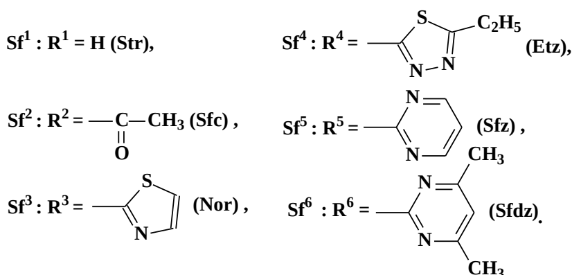
Figura 2. Schema de sinteză a compușilor coordinativi VII-XII
